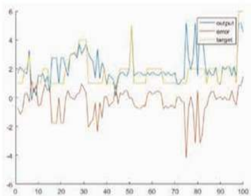
Fig.(5).PredictedOutputvsErrorsvsActualOutput
